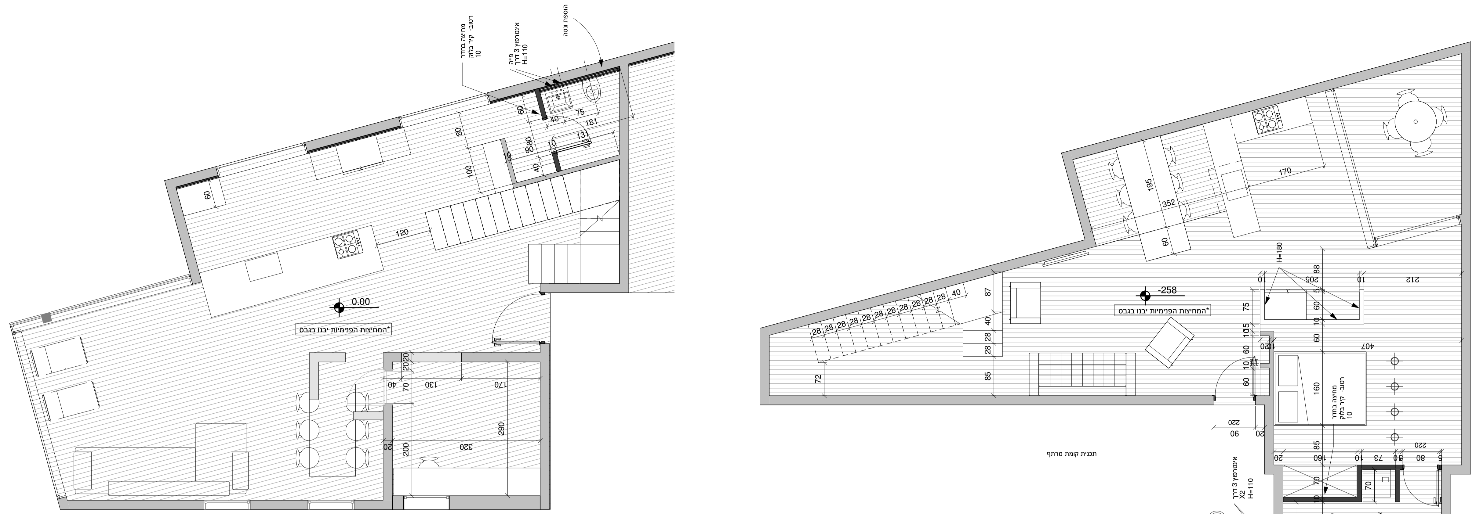
תוכנית קומה ראשונה
